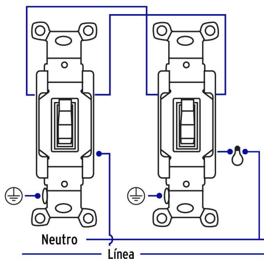
Diagrama de conexión
