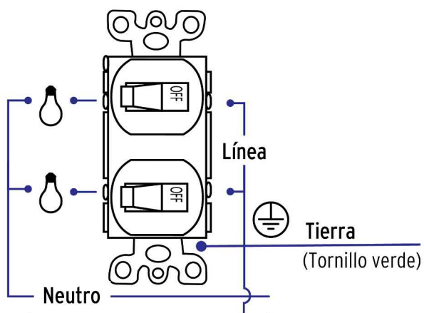
Diagrama de conexión
